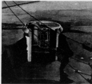
Brønnhode i silo i havbunnen – Første gang anvendt av Saga i feltutbygging på Tordis-feltet i 1993.
