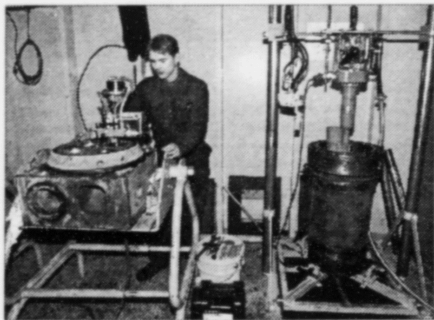
Terji Holm Jacobsen klárar at slípa toppstykkið hjá grønlandska trolararnum Sisimiut, meðan maskinan við síðuna av slípar fódringina samstundis.
