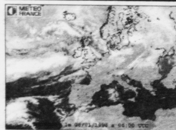
Eitt lágrýst sunnan fyri Ísland stendur næstan í stað, og eitt nýtt lágrýst í ein útsynning úr Íslandi gongur í ein landnyring og dýpst.
