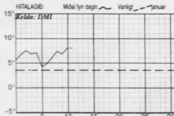
Hitalagið málit frá 13/01, kl 06 00 -14/01, kl 06 00 . Hitin í gjár: 5,7°C Minsti hiti máldur í jan.: -8,8° Hægsti hiti máldur í jan.: 11,6°
