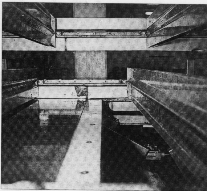
Soleiðis sær »fallemmurin« út. Tá fiskurin er vígaður greiðir skipanin frá íggjøgnum hvat portur fiskurin skal og tá fiskurin kemur hartil, so fer lemmurin upp og fiskurin dettur niður í kassan. Síðan letur portrið aftur og letur ikki upp aftur fyrr enn næsti fiskurin skal íggjøgnum
