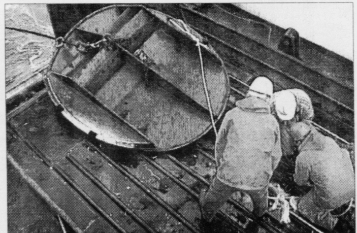
Á myndini sæst nýggi lemmurin, sum Helgi Larsen hevur upfunnið. Tað snilda við lemmunum er, at tógmeið ikki nýtist at vera so stór
