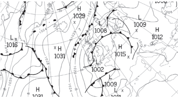
Hátrýstið í útsynning úr Íslandi viknar nakað. Lágtrýstið sunnan fyrri Írland fer suðureftir.
