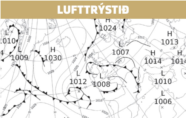
Eitt hátrýst, 1030 hPa. í útsynning úr Íslandi stendur mestsum í stað.
