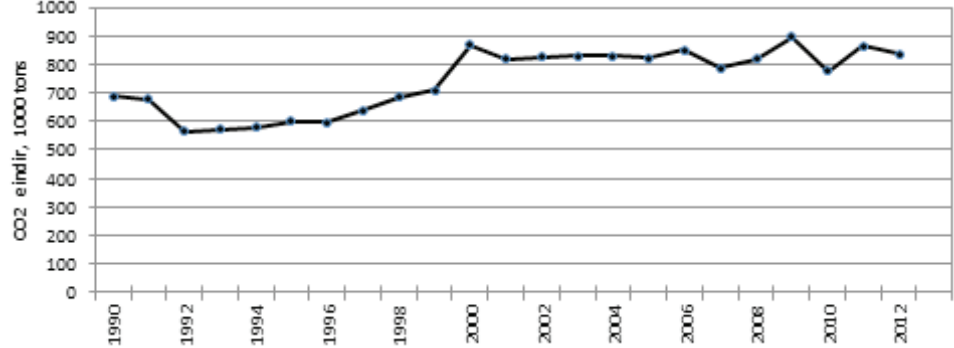
Samlaða útláti av vakstrarhúsgassi, 1990 til 2013
