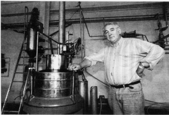
– Tað gongur skjótt fyrri seg á lýsivirkinum. Tað er bara eitt korter frá tí, at livurin fer í damparan, til lýsið verður kolt aftur. Her stendur Jógvan á Húsamørk við sentrifuguna
