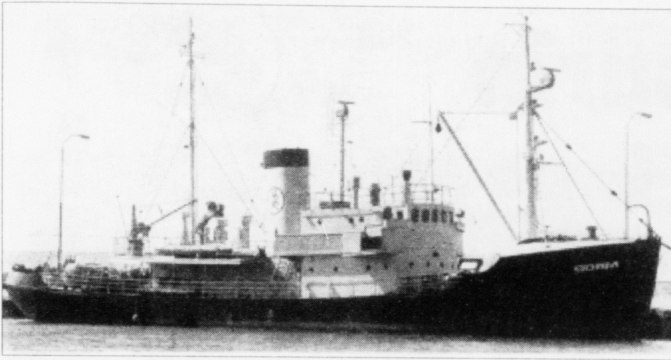
»Gorm« er bjargingskip, heimahoyrandi í Hanstholm, og sambært Dansk Illustreret Skibsliste er hann bygdur á Nakskov Skibsværft í 1944. Hann er 321 brt., 39 metrar langur og góðar 8 metrar breiddur. Skipið er höfuðsumvælt í 1972, siglir 12 mál
