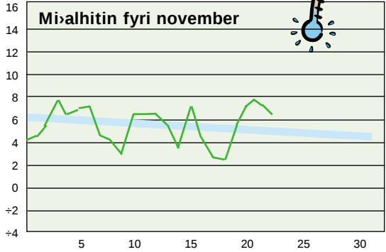
Hítalagið mált frá 23/11 kl. 06 00 –24/11 kl. 06 00 . Hitin í gjár: 6,4° Minsti hiti máldur í nov.: +7,2° Mesti hiti máldur í nov.: 12,2°
