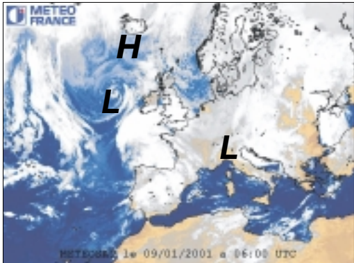
Hátrýstið sunnan fyri Ísland fer í landsynn- ing.
