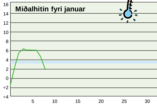
Hitalagið mált frá 08/01 kl. 06 00 –09/01 kl. 06 00 . Hitin í gjár: 1,9° Minsti hiti máldur í jan.: +8,8° Mesti hiti máldur í jan.: 11,6°
