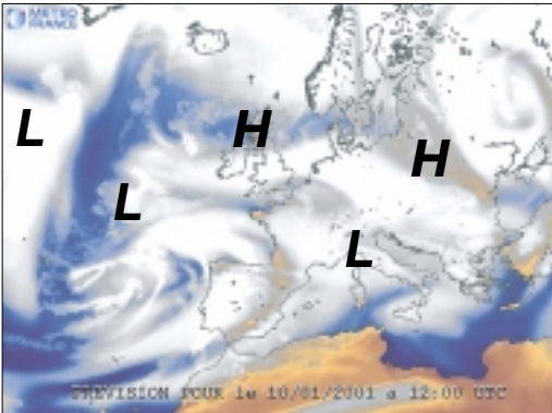
Eitt lágtrýst tekur seg upp yvir Atlantshavi- num á umleið 50N-30V og fer í landnyrðing og dýpist.
