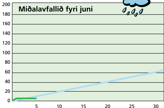
Avfallið: 2,0 mm – mált frá 4/6 kl. 06 00 – 5/6 kl. 06 00 Avfallið higartil í juni: 3,0 mm
