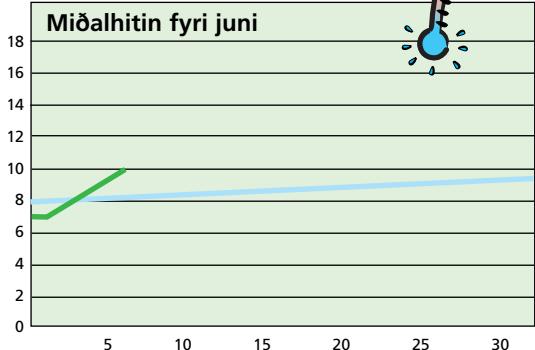
Hitalagið mált frá 4/6 kl. 06 00 – 5/6. 06 00 . Hitin í gjár: 9,0° Minsti hiti máldur í juni: 0,0° - Mesti hiti máldur í juni: 20,0°
