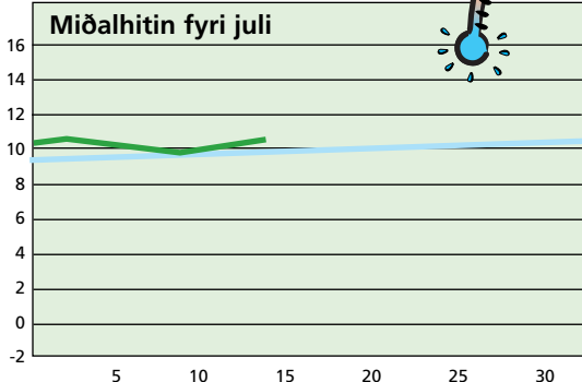
Hitalagið mált frá 13/07 kl. 06 00 – 14/07 06 00 . Hitin í gjár: 9,9° Minsti hiti máldur í juli: 0,4° - Mesti hiti máldur í juli: 20,2°
