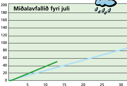
Avfallið: 3,0 mm – mált frá 13/07 kl. 06 00 – 14/07 06 00 . Avfallið higartil í juli: 51 mm
