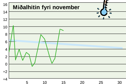
Hitalagið mált frá 14/11 kl. 06 00 –15/11 kl. 06 00 . Hitin í gjár: 8,9° Minsti hiti máldur í nov.: +7,2° Mesti hiti máldur í nov.: 12,2°
