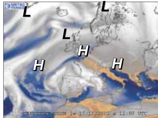
Lágtrýstið í útsynning úr Føroyum fer í landnyrring og verður yvir Føroyum sunnunáttina. Háttrýstið í útsynning úr Írlandi breiðir seg móti Føroyum í næstu viku.
