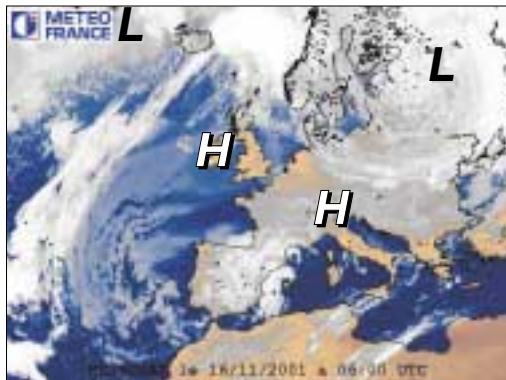
Eitt lágtrýst, 986 hPa. yvir Grønlandsfjørðinum fer skjótt í landnyrring.
