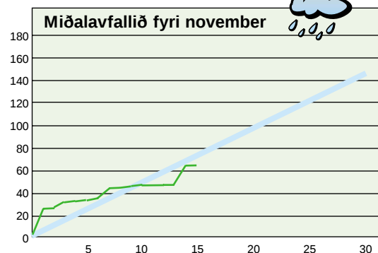
Avfallið: 0,2 mm – mált frá 14/11 kl. 06 00 –15/11 kl. 06 00 Avfallið higartil í november: 65,4 mm
