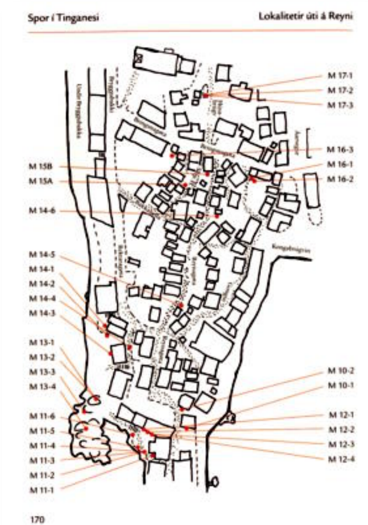
Kort yvir lokalitetir úti á Reyni
