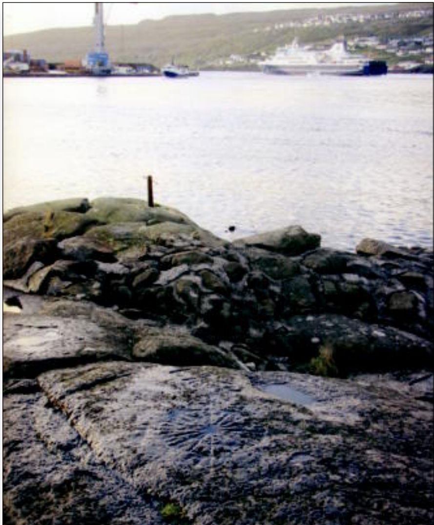
Sólurið á tí fløtu helluni vestantil á Nesinum
